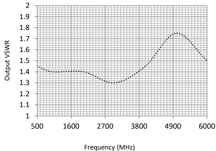
Output VSWR
