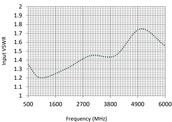
Input VSWR
