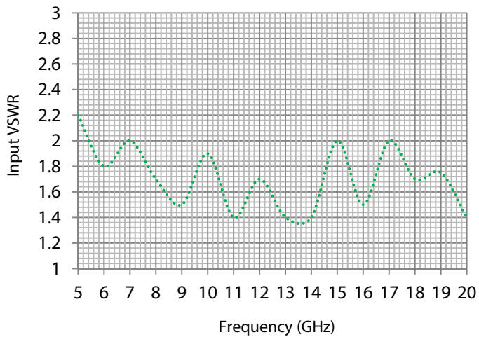
Input VSWR
