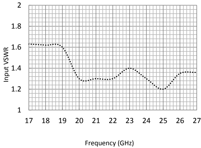
Input VSWR
