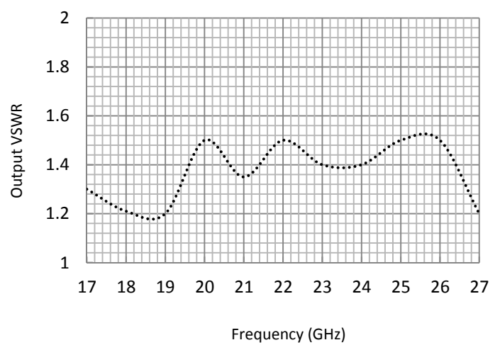
Output VSWR
